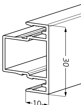
Tussenprofiel
