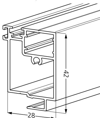
Deurprofiel
